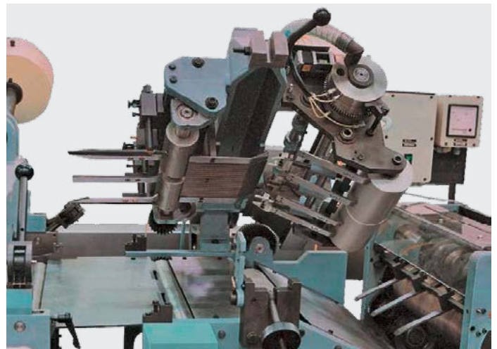
Faltstation – eingerichtet für Klotzbodenfertigung
