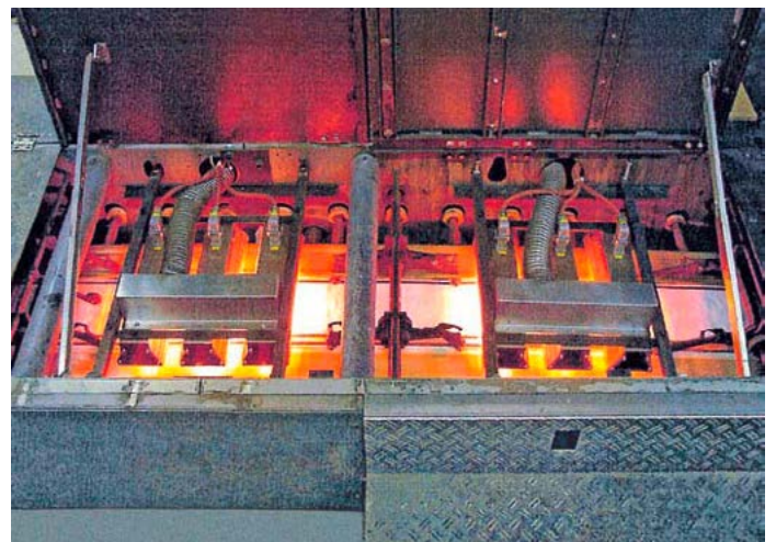
Neues IR-Trocknung-Retrofit
